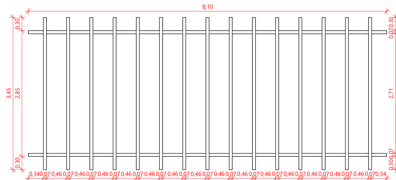
6 Planta de detalhe - Pergolado ESC.: 1 : 50
