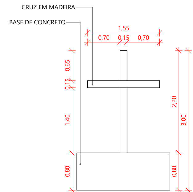
2 Elevação frontal ESC.: 1 : 50
